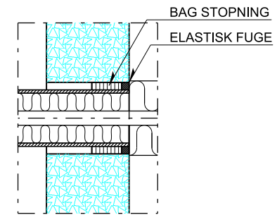
DETALJE A, 1:5
